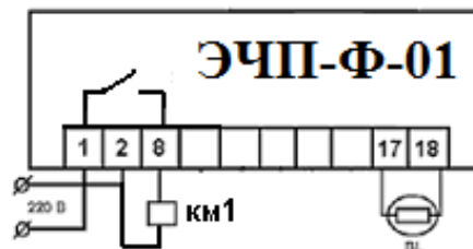
Рис 2. Схема включения программатора ЭЧП-Ф-01
